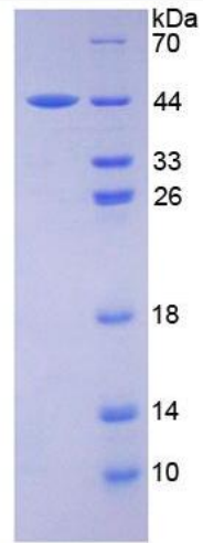
15% SDS-PAGE
