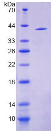
SDS-PAGE
