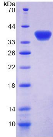
SDS-PAGE
