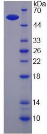
15% SDS-PAGE
