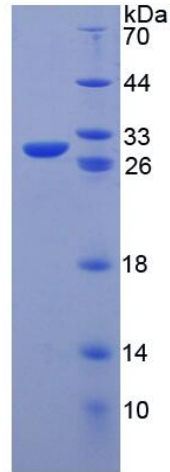
15% SDS-PAGE
