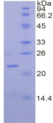
15% SDS-PAGE
