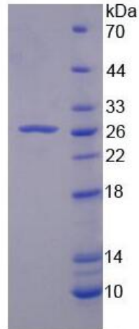
15% SDS-PAGE
