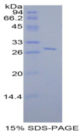
15% SDS-PAGE
