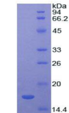
15% SDS-PAGE
