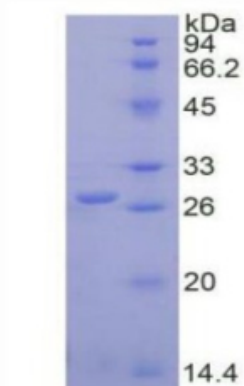
15% SDS-PAGE
