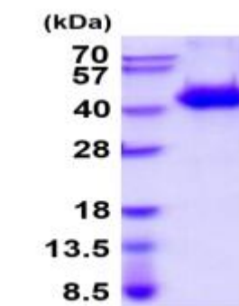
15% SDS-PAGE (3μg)
