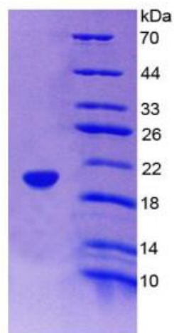
15% SDS-PAGE
