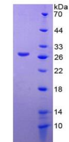
15% SDS-PAGE
