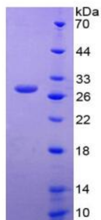
15% SDS-PAGE
