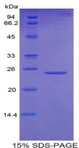
15% SDS-PAGE
