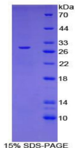
SDS-PAGE
