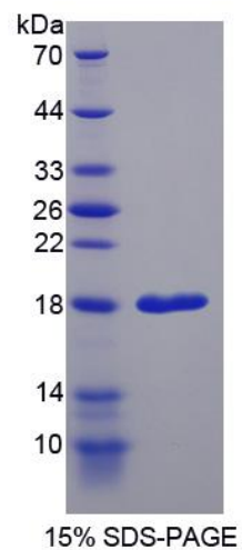
SDS-PAGE
