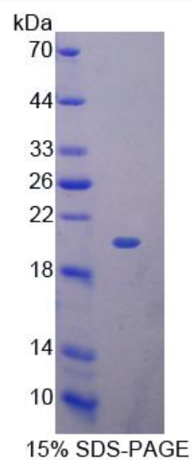
SDS-PAGE
