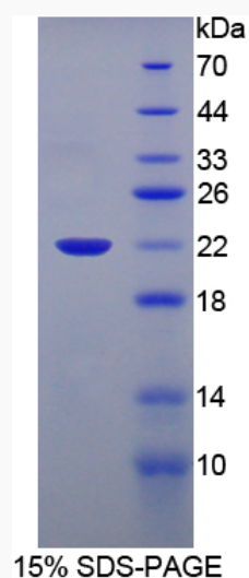
SDS-PAGE
