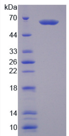
15% SDS-PAGE
