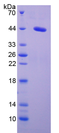
SDS-PAGE
