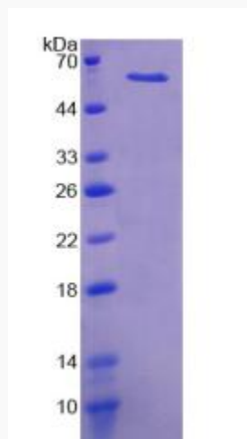
SDS-PAGE
