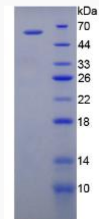
SDS-PAGE
