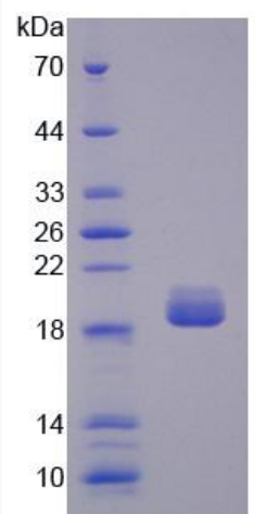
15% SDS-PAGE
