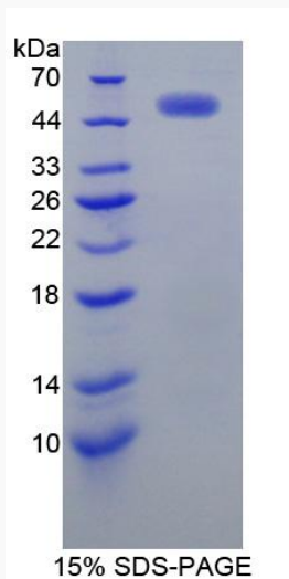
SDS-PAGE
