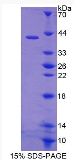
SDS-PAGE
