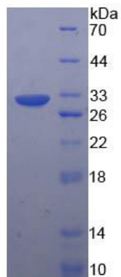
15% SDS-PAGE
