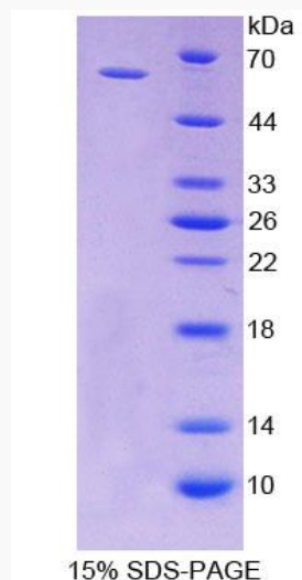
SDS-PAGE
