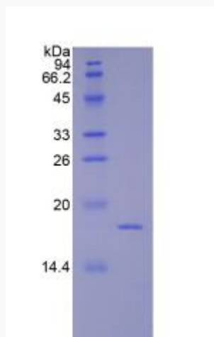
SDS-PAGE
