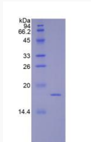
SDS-PAGE
