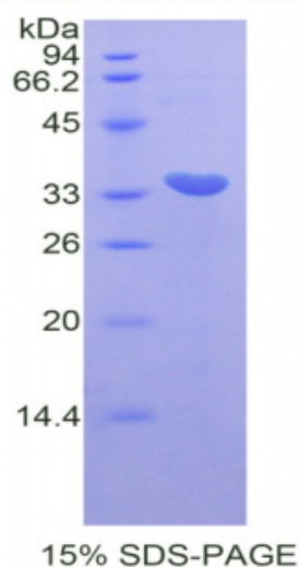
SDS-PAGE
