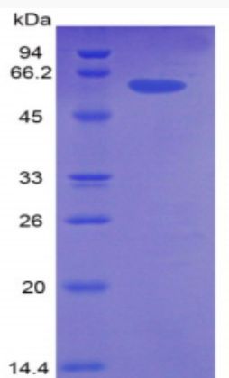
15% SDS-PAGE
