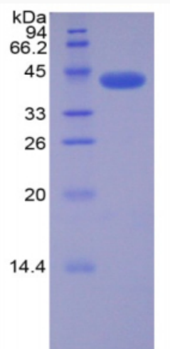
15% SDS-PAGE
