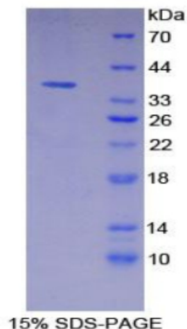
SDS-PAGE
