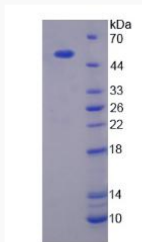
SDS-PAGE
