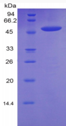
15% SDS-PAGE
