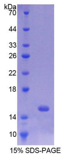
SDS-PAGE
