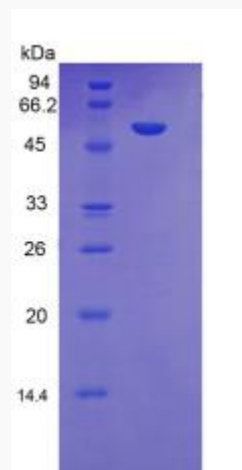
SDS-PAGE
