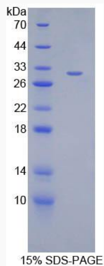
SDS-PAGE
