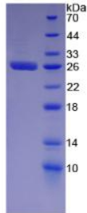
SDS-PAGE
