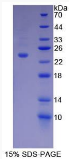
SDS-PAGE
