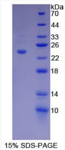
SDS-PAGE
