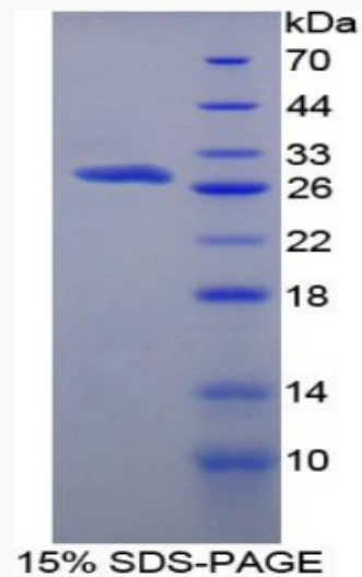
SDS-PAGE
