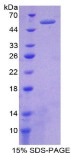
SDS-PAGE
