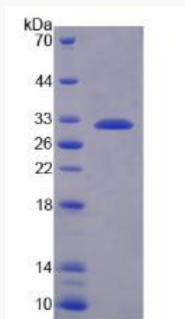
SDS-PAGE
