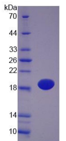
SDS-PAGE
