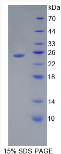
SDS-PAGE
