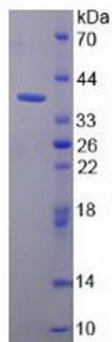
SDS-PAGE
