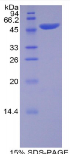
SDS-PAGE
