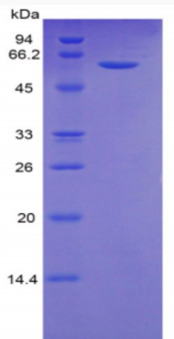
15% SDS-PAGE
