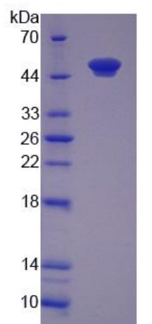
15% SDS-PAGE
