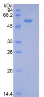
15% SDS-PAGE
